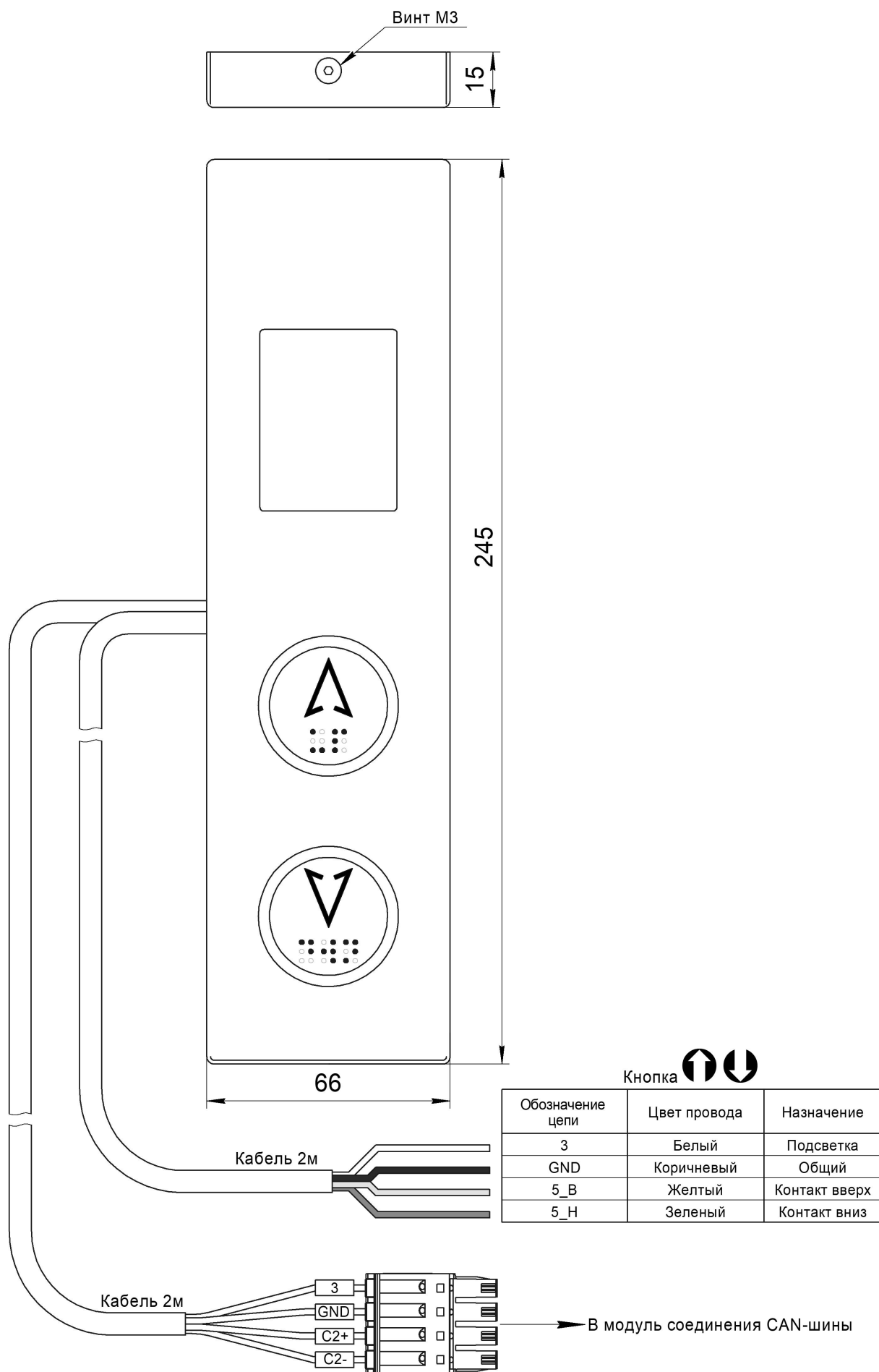
Рис.1 Внешний вид, габаритные и установочные размеры Вызывного поста ВП-2103-1086-09
